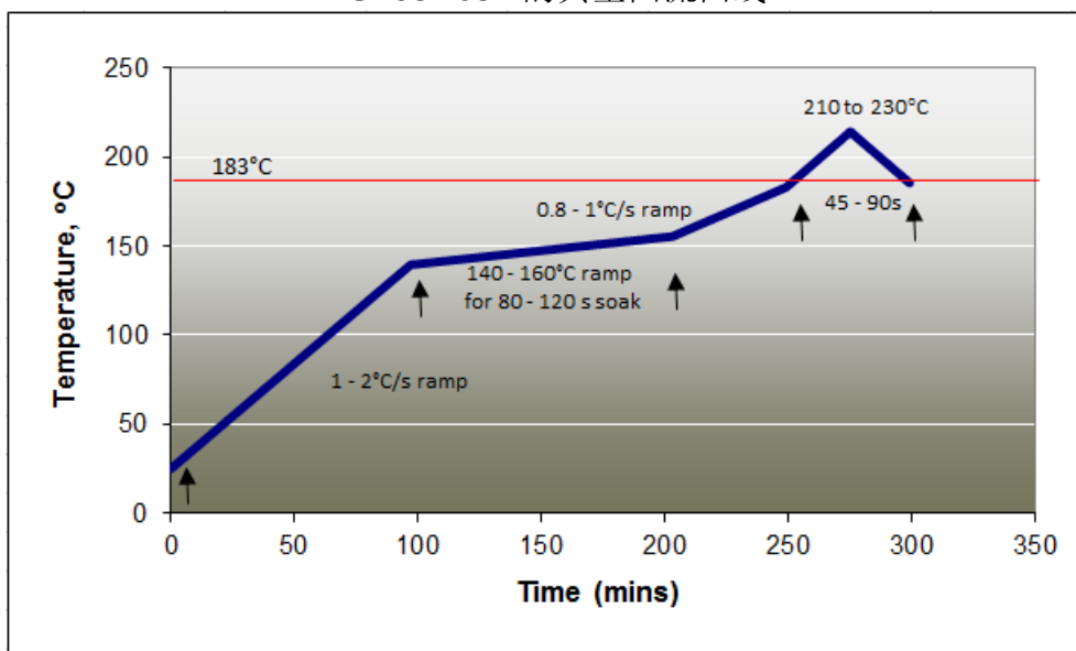
图表 2. Alpha-Fry™ EGP-120 Sn63Pb37 的典型回流曲线
