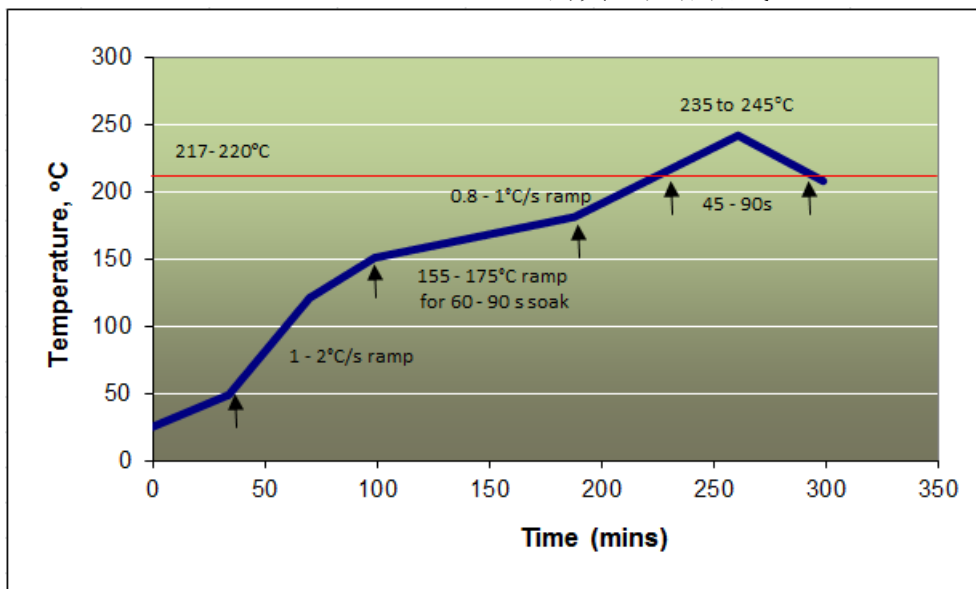
图表 1. Alpha-Fry™ EGP-120 SAC305 & SAC 0307 的典型回流曲线
